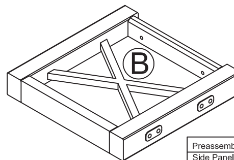
SIDE FRAME MARCO CADRE T5045096020EL Qty/Qty/Qté: 2
