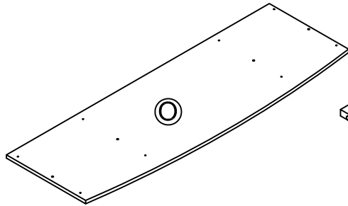
BOTTOM PANEL Panel base PANNEAU INFÉRIEUR T1807096150CS
