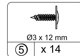
SCREW Tornillo VIS TCS1048
