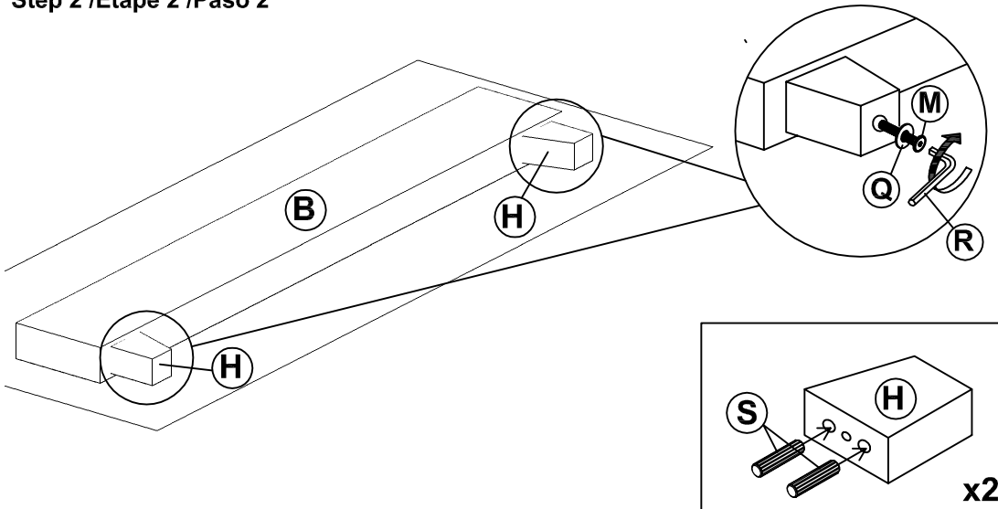
Step 2 /Étape 2 /Paso 2
