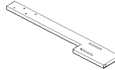
x1 RD365-250-1-LEGR Headboard legs (right) * Pattes de la tete de lit (droite) Pattes de cabecera (derecha)
