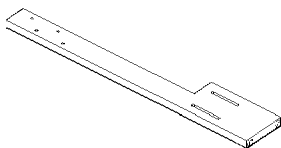
x1 RD365-270-1-LEGL Headboard legs (left) * Pattes de la tete de lit (gauche) Pattes de cabecera (izquierda)
