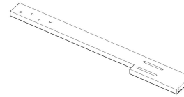
x1 R2534-250-208-LEGR Headboard leg (Right) * Pattes de la tete de lit (droite) Pattas de cabecera (derecha)
