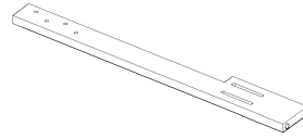
x1 R2534-250-208-LEGL Headboards leg(left) * Pattes de la tete de lit (gauche) Pattas de cabecera (Izquierda)
