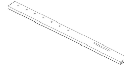
x1 RD307-650-HLEG2 Headboard legs (Left) * Pattes de la tete de lit (gauche) Pattas de la cabecera(Izquierda)
