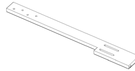
x1 R2534-270-208-LEGR Headboard leg (Right) * Pattes de la tete de lit (droite) Pattas de cabecera (derecha)
