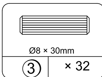
WOOD DOWEL TLW8030
